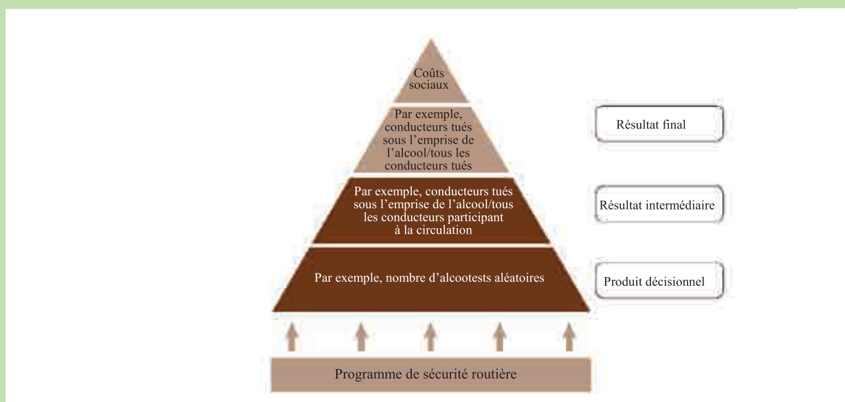
Figure 3. Hiérarchie des objectifs de sécurité routière pour la conduite sous l'emprise de l'alcool 9
